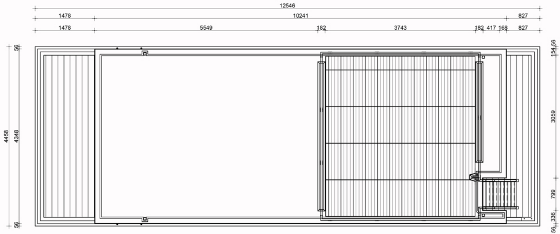
GRUNDRISS OBERDECK
