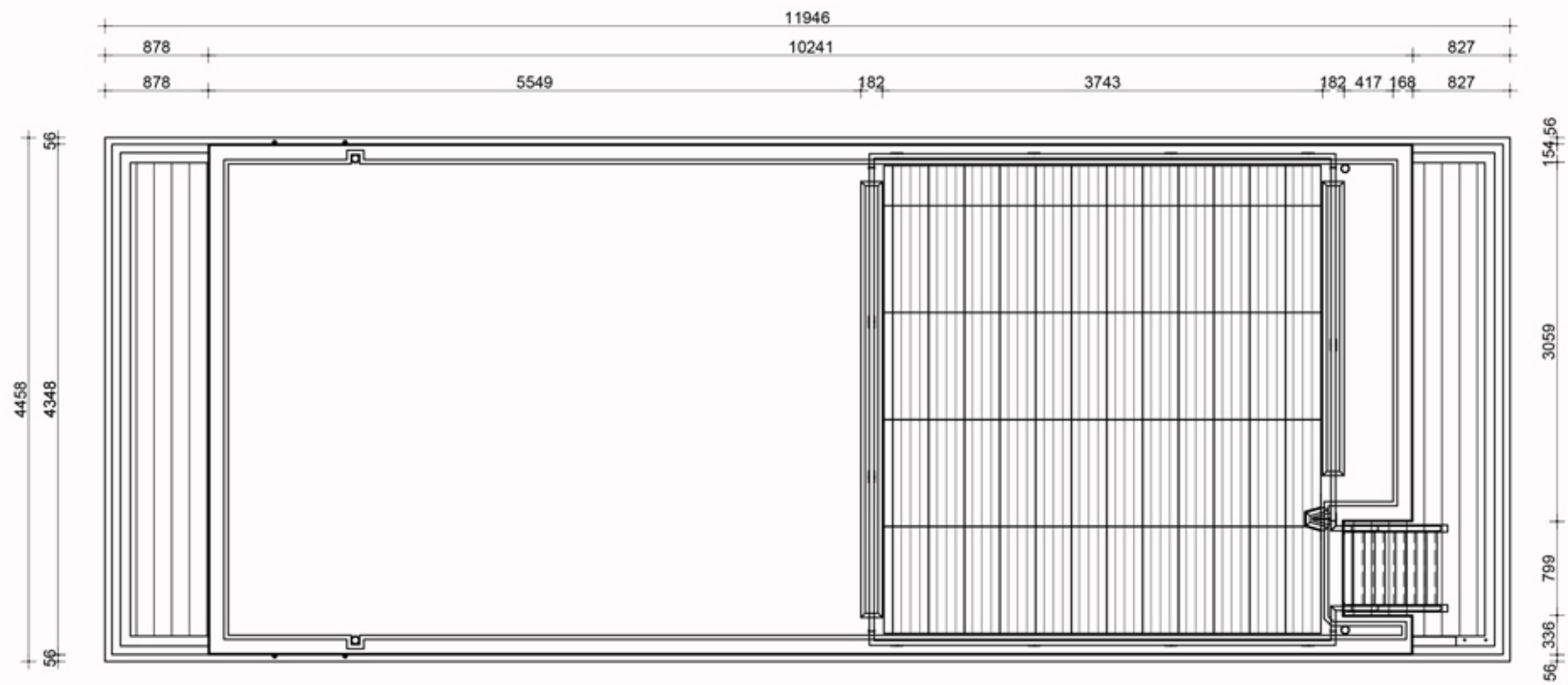
GRUNDRISS OBERDECK
