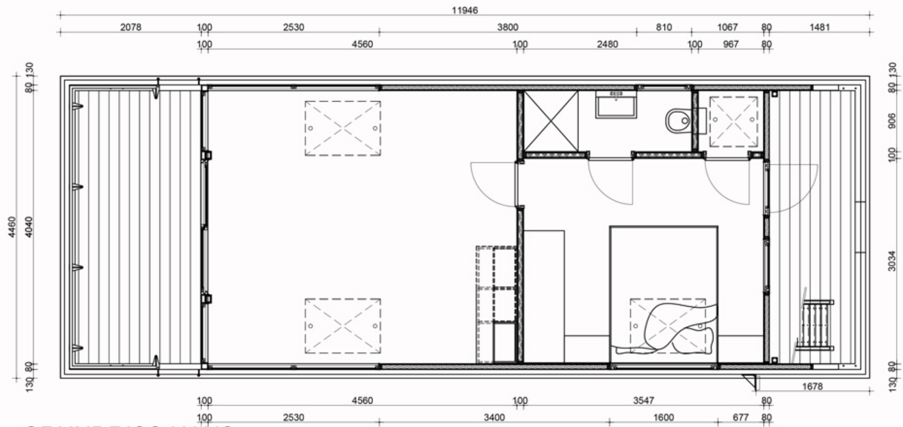
GRUNDRISS HAUS
